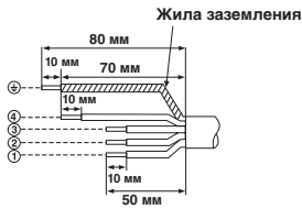
Оголение конца соединительного кабеля
